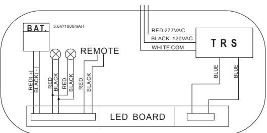
COMBO RC Wiring Diagram:
