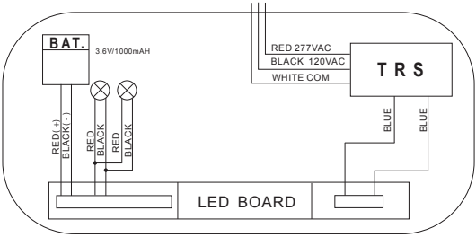
COMBO Wiring Diagram:
