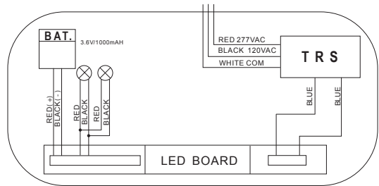
COMBO Wiring Diagram:
